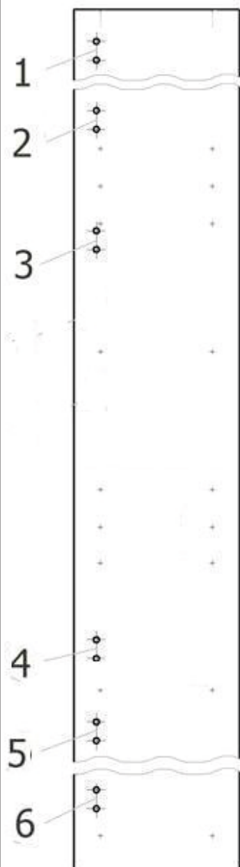
Схема расположения отверстий под петли на дет.№ 1173
