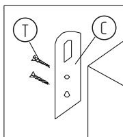
Крепление подбески (комплект №20)
