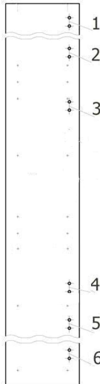
Схема расположения отверстий под петли на дет. №1174
